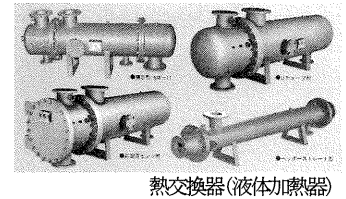
熱交換器(液体加熱器)
